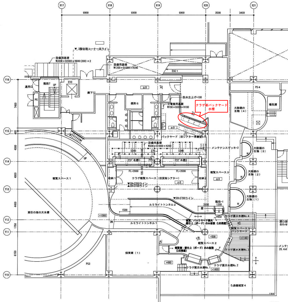
平面図
