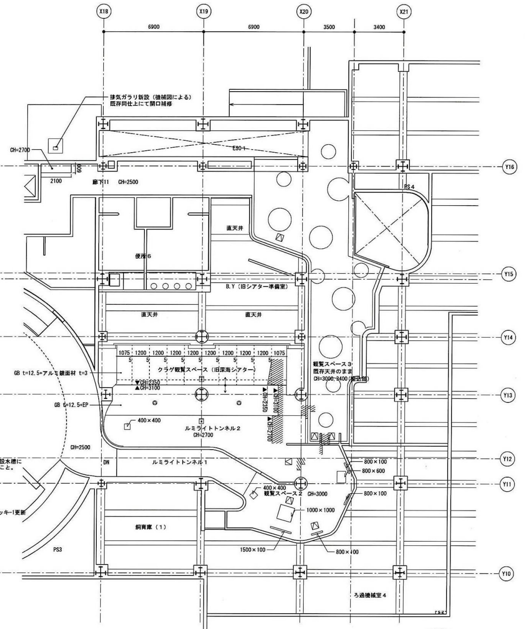
天井伏図
