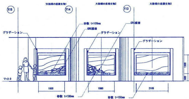
大陸棚の生物 1 ～ 3 立面図 S=1:50
